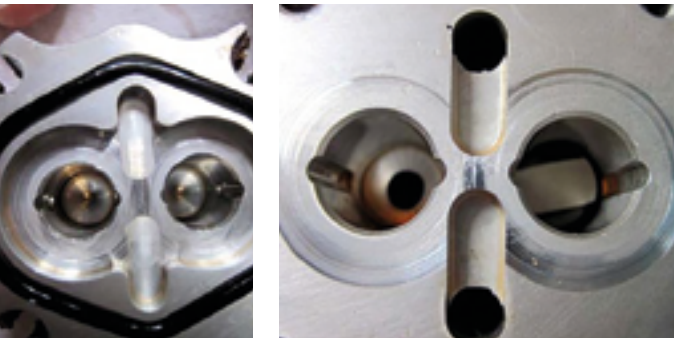
Usure prématurée dans un corps et des engrenages d'une pompe d'engrenages externes.
