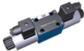
CETOP 3 (NG-6) SERIE VNKPV-6 PROPORCIONAL .MAX BAR 315 30 l/min. PROPORTIONAL CETOP 3 (NG-6) SERIE 4VNKPV-6 MAX.P 315 BAR 30 L/MIN. CETOP 3 (NG-6) SÉRIE 4VNKPV-6 PROPORTIONNEL MAX BAR 315 30 l/min.
