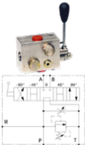
DISTRIBUIDORES MANUALES ROTATIVOS PARA VNKP/VNKR CON LIMITADORA Y REGULADOR DE CAUDAL CUERPO ALUMINIO MANUAL ROTARY DIRECTIONAL CONTROL VALVE VNKP/VNKR WITH RELIEF AND FLOW CONTROL VALVE ALUMINIUM BODY DISTRIBUTEURS À MAIN ROTATIFS VNKP/VNKR AVEC LIMITEUR ET RÉGULATEUR DE DÉBIT CORPS ALUMINIUM
