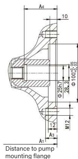
Section A-B
