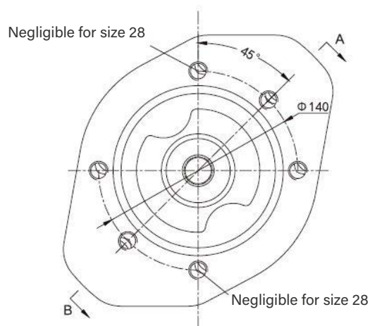
Section A-B
