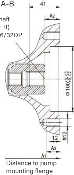
Section A-B
