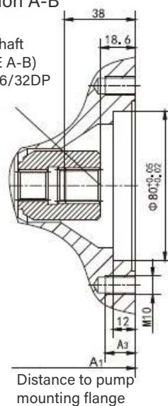
Section A-B
