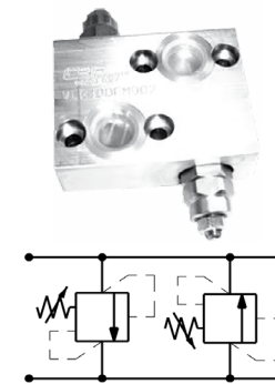
LIMITADORAS DOBLE PARA VNKS 300 BAR CUERPO ALUMINIO DOUBLE RELIEF VALVES VNKS 300 BAR ALUMINIUM BODY LIMITEURS DOBLES POUR VNKS 300 BARS CORPS ALUMINIUM
