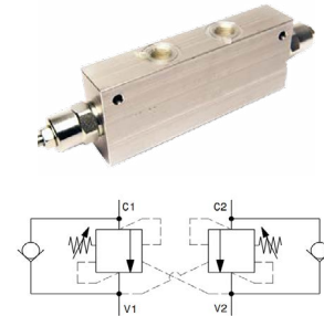
OVERCENTER DOBLE 350 BAR CUERPO ALUMINIO DOUBLE OVERCENTER 350 BAR ALUMINIUM BODY VALVE D'ÉQUILIBRAGE DOUBLE 350 BAR CORPS ALUMINIUM
