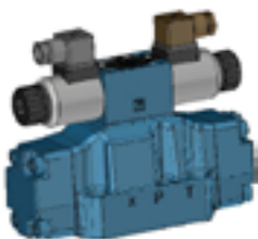
CETOP 8 (NG-25) VNKEH-25 P. MAX. 315 BAR 500 l/min. CETOP 8 (NG-25) VNKEH-25 P. MAX. 315 BAR 500 L/MIN. CETOP 8 (NG-25) VNKEH-25 P. MAX. 315 BAR 500 l/min.
